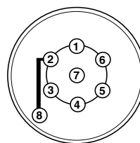
Collegamento dei cavi alla presa a 7 poli
