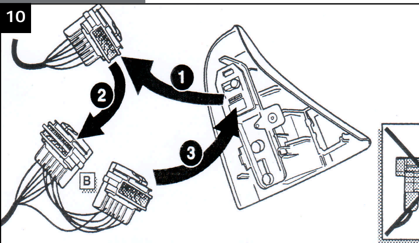
10 RECHTEN HECKLEUCHTESATZ FEU ARRIERE DROIT RIGHT REARLIGHT UNIT RECHTER ACHTERLICHT
