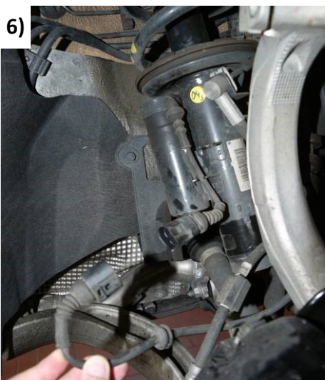
6) Steckverbindung lösen.
