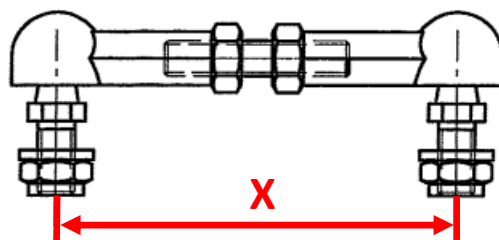
Abb. 1: Einstellmaß X HA
