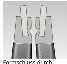
Formschluss durch Verpressung
