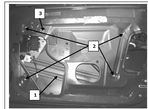
Porta lato destro, Portière avant droite, Right front door, Puerta lado derecho, Vorne rechte Tür, Porta frente dijeta, Sag on kapi, νότια εμπρόσθια δεξιά
