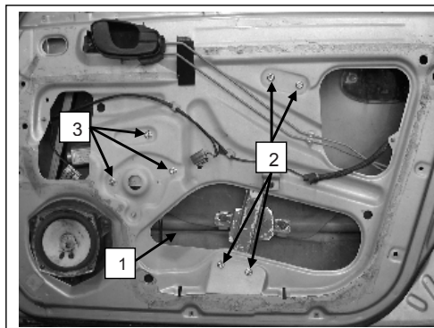
Porta lato destro, Portière avant droite, Right front door, Puerta lado derecho, Vorne rechte Tür, Porta frente diarieta, Sag on kapi, норта смпроста десја
