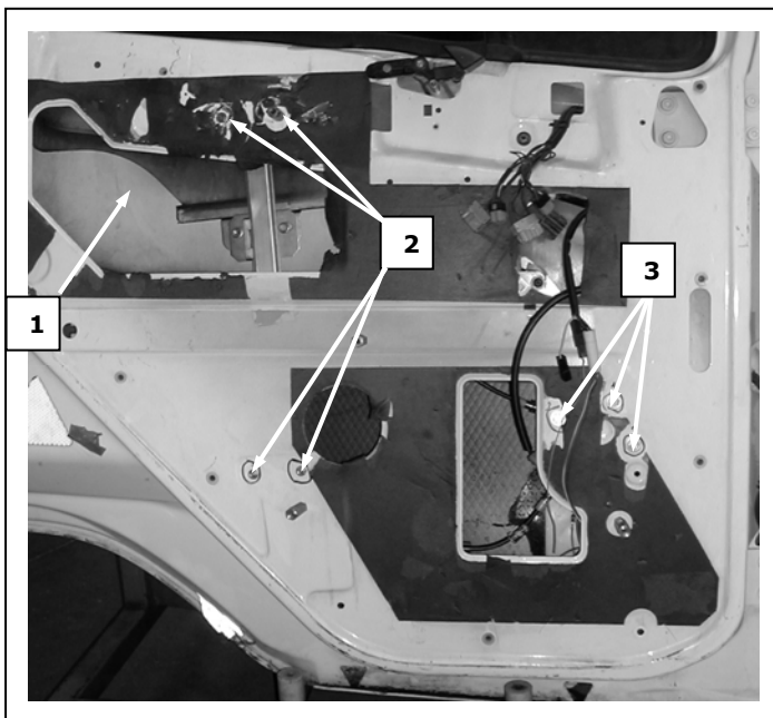
Porta lato sinistro, Portière avant gauche, Left front door, Puerta lado izquierdo, Vorne links Tür, Porta frente esquerda, Sol on kapi, πόρτα εμπρόςα αριστερή
