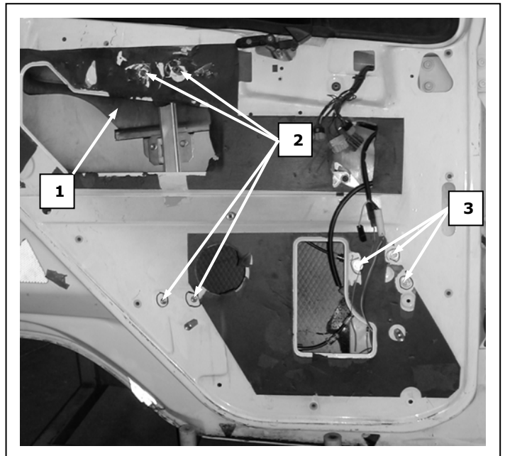
Porta lato sinistro, Portière avant gauche, Left front door, Puerta lado izquierdo, Vorne links Tür, Porta frente esquerda, Sol on kapi, πόρτα εμπρός/αριστερή
