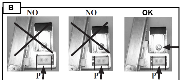
Porta lato destro, Portière avant droite, Right front door, Puerta lado derecho, Vorne rechte Tür, Porta frente dirieta, Sag on kapı, πόρτα εμπρόςθια δεξιά
