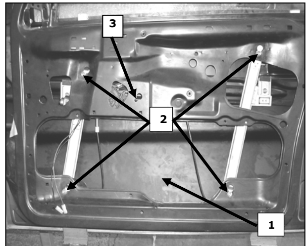
Porta lato destro, Portière avant droite, Right front door, Puerta lado derecho, Vorne rechte Tür, Porta frente dirieta, Sag on kapı, πόρτα εμπρόςθια δεξιά
