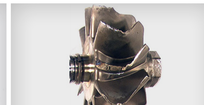
Rupture par fatigue de la roue de turbine en raison d'une vitesse cyclique trop élevée
