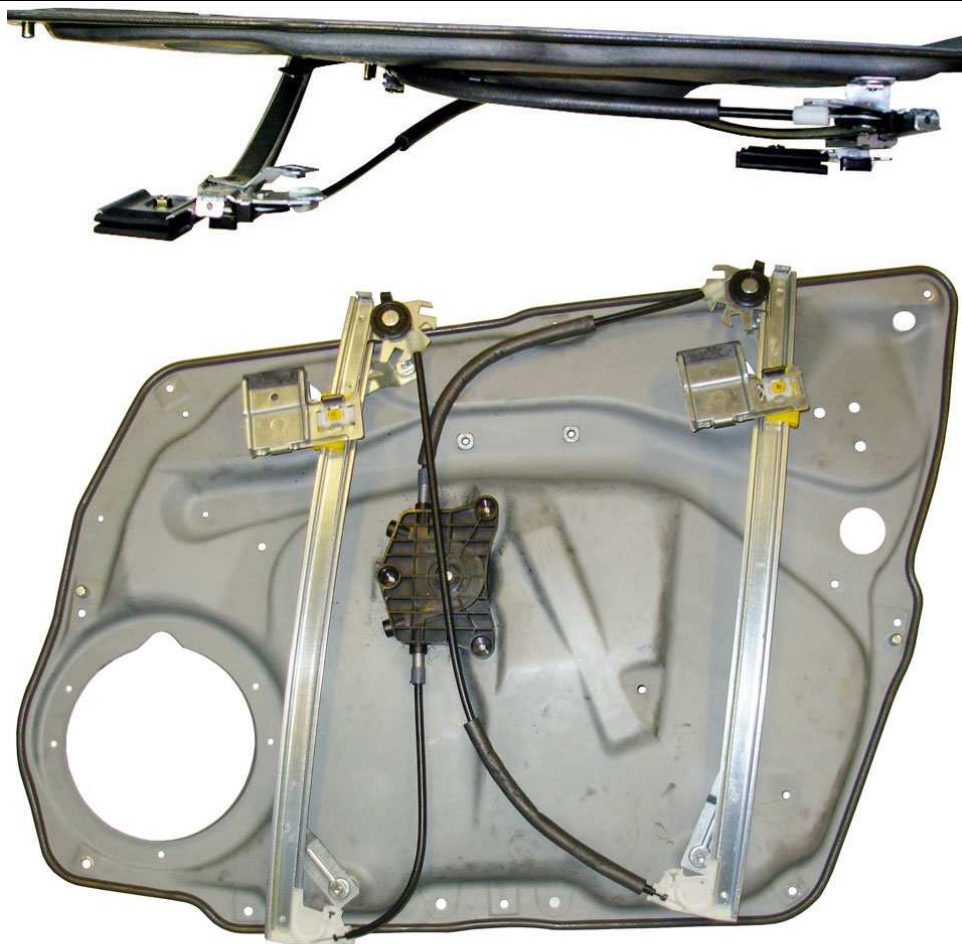
POWER WINDOW LEFT ALZACRISTALLI ELETTRICO SX
