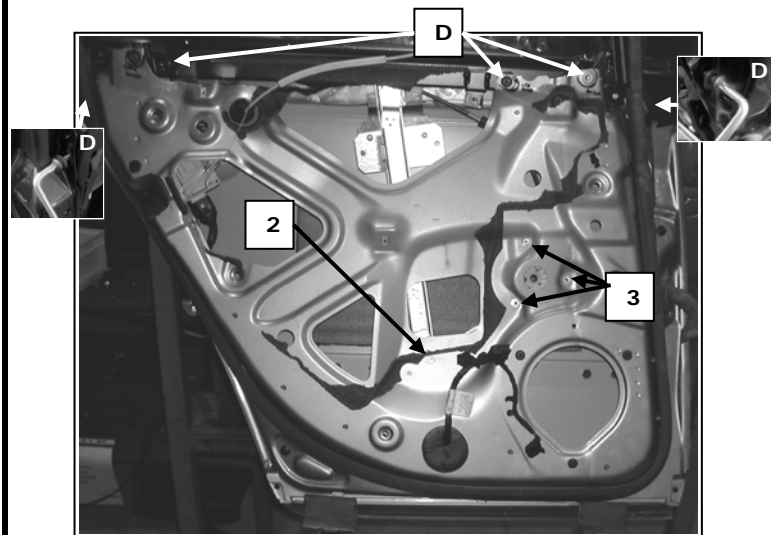
Puerta lado derecho, Right rear door
