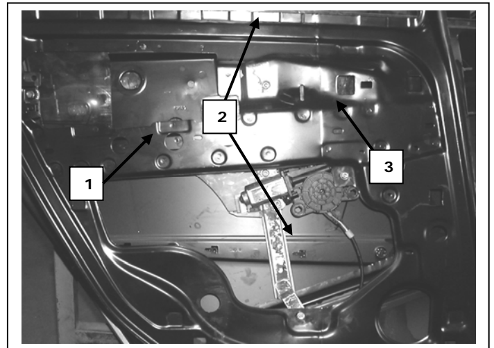
Puerta lado izquierdo, Left rear door
