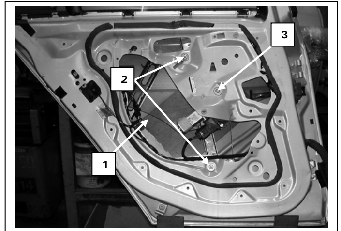
Puerta lado izquierdo, Left rear door
