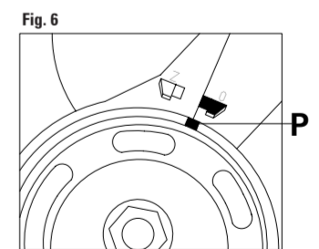
FIGURA 5 Verificar la correcta alineación de la marca de puesta en fase O. FIGURA 6 Verificar la correcta alineación de la marca de puesta en fase P.
