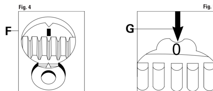
FIGURA 4 Segni di riferimento sul volano: verificare il corretto allineamento delle tacche di fase F.
