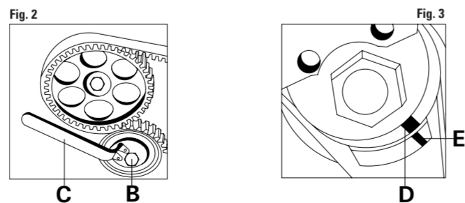
FIGURA 2 Allentare il bullone di bloccaggio B e ruotare in senso orario il tendicinghia utilizzando la chiave C agendo sull'eccentrico di registro.
