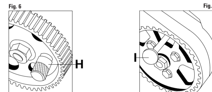
FIGURA 6 Inserire l'apposito attrezzo di bloccaggio della puleggia della pompa di iniezione H.
