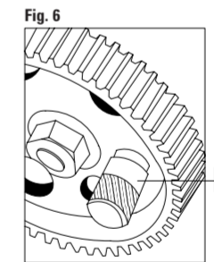
FIGURA 6 Insertar la herramienta para inmovilización de polea de bomba de inyección H. FIGURA 7 Insertar la herramienta para inmovilización de polea de bomba de inyección I. FIGURE 6 Introduire l'outil approprié de blocage poulie pompe d'injection H. FIGURE 7 Introduire l'outil approprié de blocage poulie pompe d'injection I.
