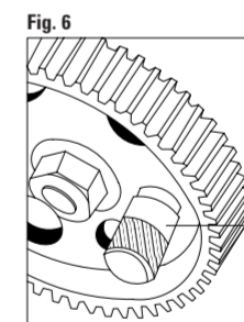
FIGURA 6 Insertar la herramienta para inmovilización de polea de bomba de inyección H. FIGURA 7 Insertar la herramienta para inmovilización de polea de bomba de inyección I. FIGURE 6 Introduire l'outil approprié de blocage poulie pompe d'injection H. FIGURE 7 Introduire l'outil approprié de blocage poulie pompe d'injection I.
