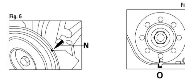
FIGURA 6 Controllare il corretto allineamento delle tacche di fase N. FIGURA 7 Controllare il corretto allineamento delle tacche di fase O.
