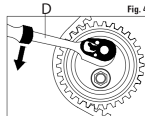
FIGURA 2: Allentare il bullone di bloccaggio del tendicinghia della distribuzione.
