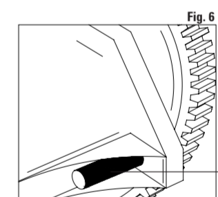
FIGURA 6: Insertar la herramienta especial para inmovilización de cigüeñal motor F, N°11 2 300.
