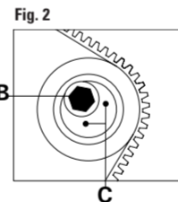
FIGURA 2 Aflojar el tornillo de fijación B, girar el tensor de correa sobre el excéntrico de regulación C en sentido contrario a las agujas de reloj hasta lograr la tensión correcta. Luego vuelva apretar el tornillo de fijación B.
