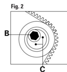
FIGURA 2 Allentare il bullone di bloccaggio B e ruotare in senso antiorario il tendicinghia sull'eccentrico di registro C fino alla corretta tensione; serrare quindi il bullone di bloccaggio B.
