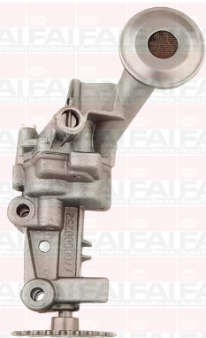
26 Teeth Sprocket
