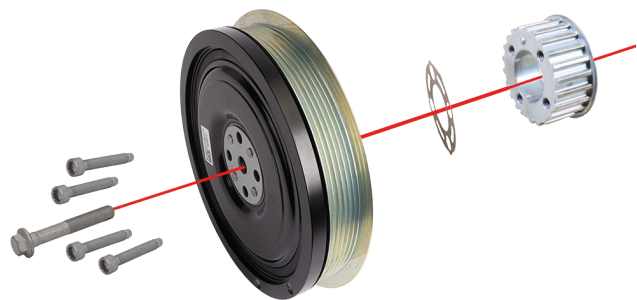
Fig. 2: Parafusos da polia desacopladora, parafuso central da cambota, polia desacopladora e anilha com revestimento de diamante.
