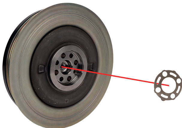
Fig. 1: Lado da cambota da polia desacopladora com anilha com revestimento de diamante. No kit mencionado, já se encontra instalado na polia desacopladora em posição de montagem.
