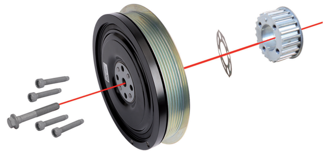
Image 2 : Vis de la poulie damper, vis centrale du vilebrequin, poulie damper et contreplaque sphérique diamantée
