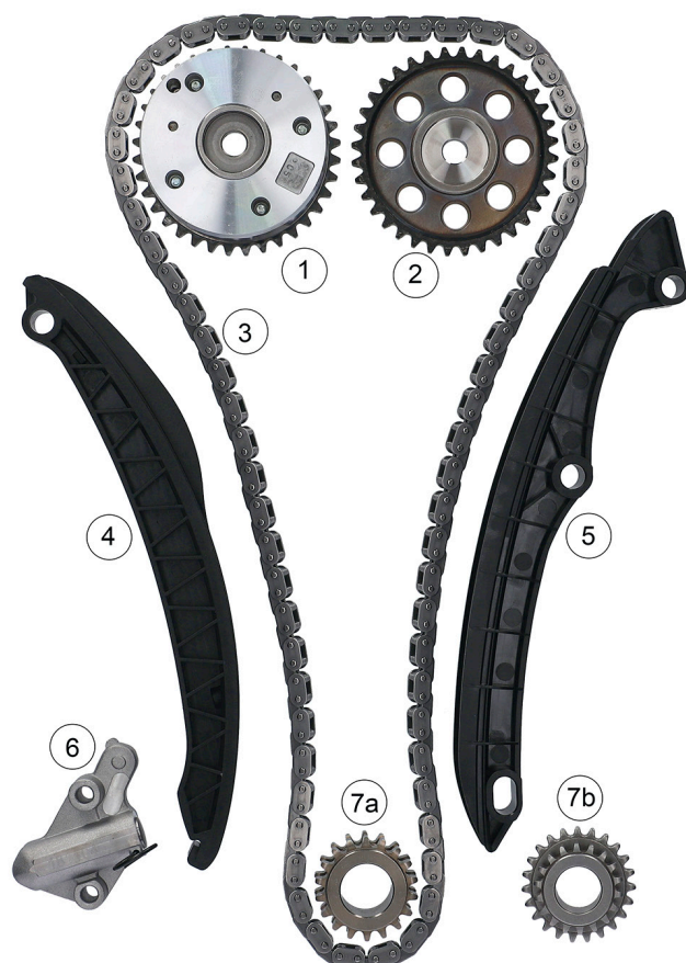
Figura 1: 559 0154 30/559 0154 31 – Componente KIT lanț de distribuție
