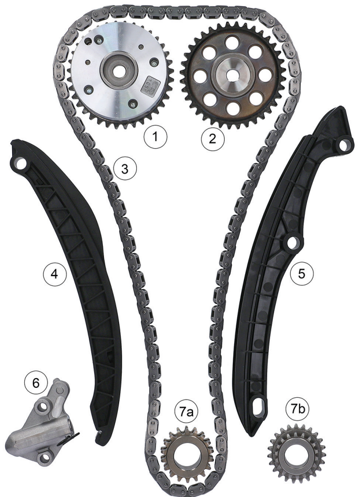
Figura 1: 559 0154 30/559 0154 31 – Componentes del kit de cadena de distribución
