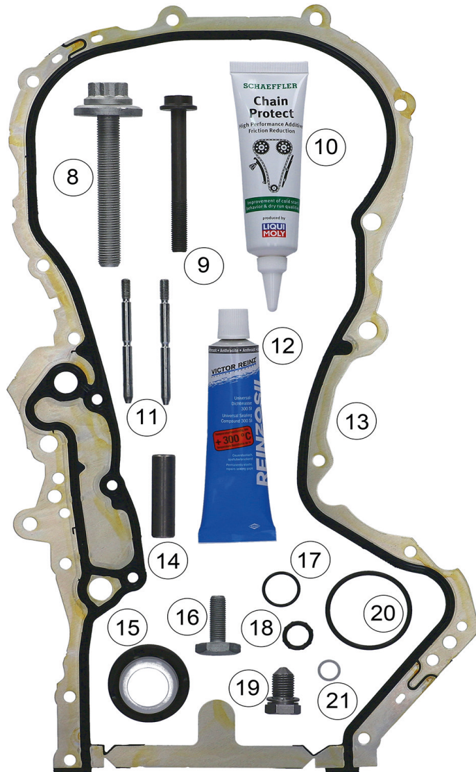
Figura 2: 559 0154 30/559 0154 31 - Accesorios del kit de cadena de distribución
