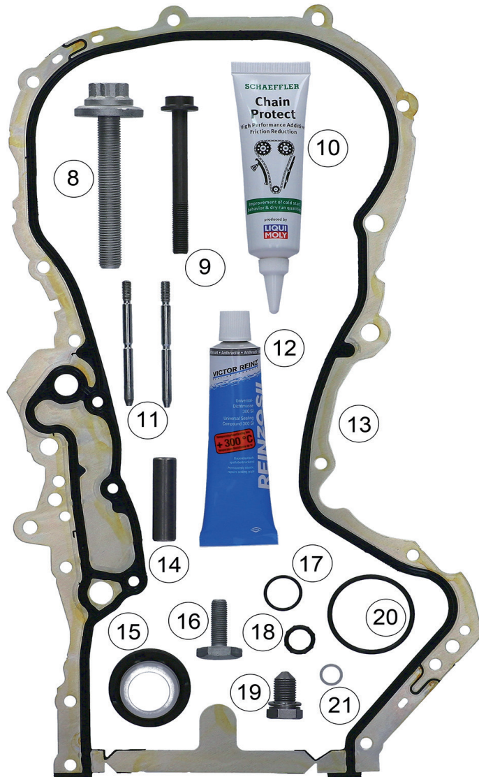
Bild 2: 559 0154 30/559 0154 31 - Anbauteile für Steuerketten-KIT
