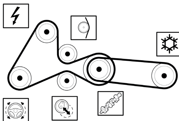
Bild 2: Hjälppaggregatdrift från motornummer 0113090 med elastisk multiribbrem
