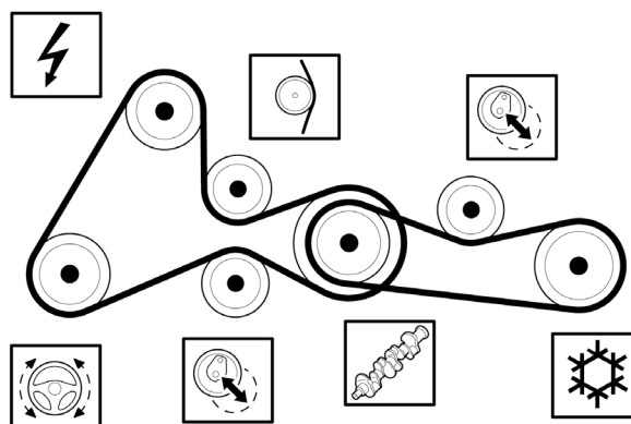
Bild 1: Hjälppaggregatdrift t.o.m. motornummer 0113089 med spännrulle
