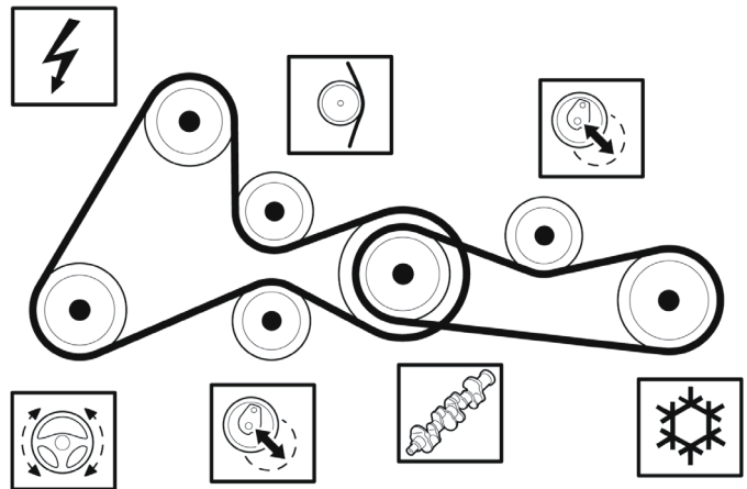
Fig. 1: Transmisión del grupo auxiliar en motores con número 0113089 o inferior con polea tensora
