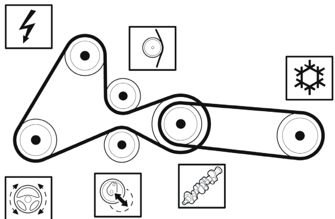
Fig. 2: Transmisión del grupo auxiliar en motores con número 0113090 o superior con correa trapezoidal elástica
