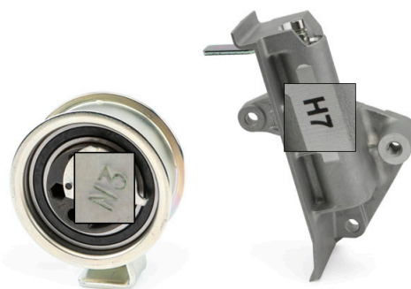
Obrázek 1: Napínací kladka 531 0396 20 s tlumičem vibrací 533 0039 10
