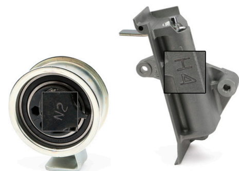
Obrázek 2: Napínací kladka 531 0436 20 s tlumičem vibrací 533 0035 10
