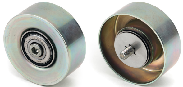
Kuva 2: 532 0398 10 – Ohjainpyörä uudella tiivistekonseptilla
