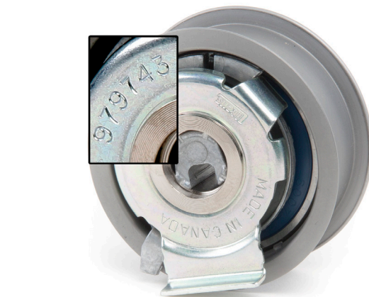
Зображення 1: 531 0777 10 – Старий натяжний ролик (979743)
