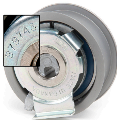
Рисунок 1: 531 0777 10 – натяжной ролик прежней конструкции (979743)
