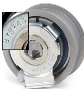
Slika 1: 531 0777 10 – Old stara remenica natezača (979743)
