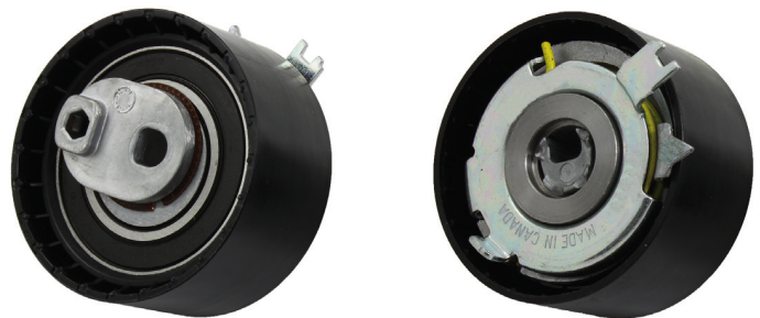
Fig. 1: Polea tensora INA 531 0710 10
