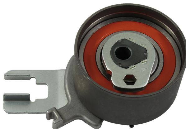
Bild 1: 531 0859 10 - spännrulle nytt utförande
