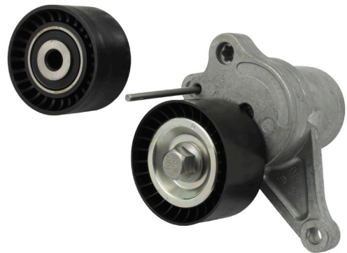
Зображення 2: Пластмасові натяжний та обвідний ролики
