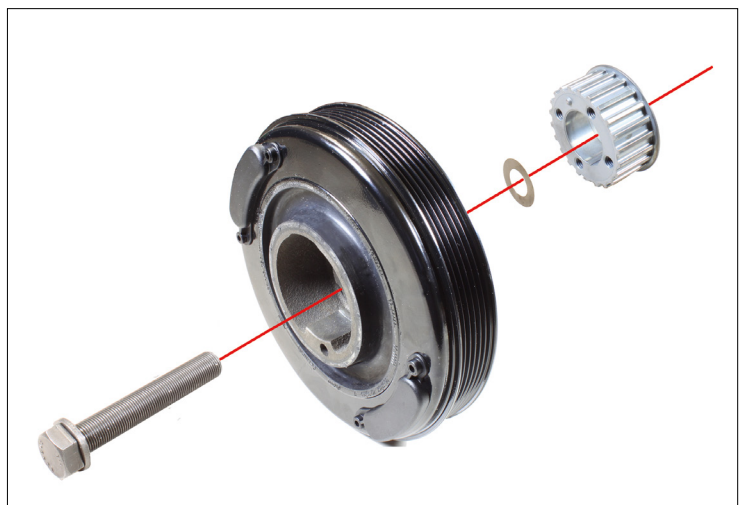
Slika 1: Ublaživač vibracija koljenastog vratila sa središnjim vijkom I dijamantnom podloškom
