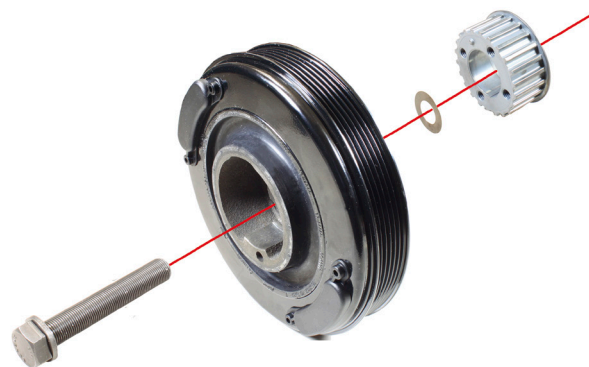
Billede 1: krumtapakselvibrationsdæmper med krumtapakselcentralbolt og diamantspændeskive
