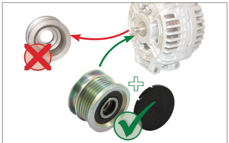
Fig. 1: Vervanging van starre rol door een dynamorijlooprool
