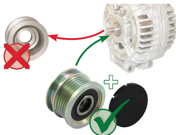
Billede 1: Udskiftning af en stiv remskive på en friløbsremskive
