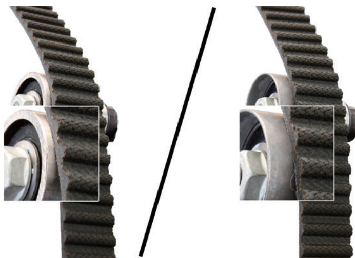
画像 2: 偏向プーリー 532 0623 10 (左) / 偏向プーリー 532 0349 10 (右)
