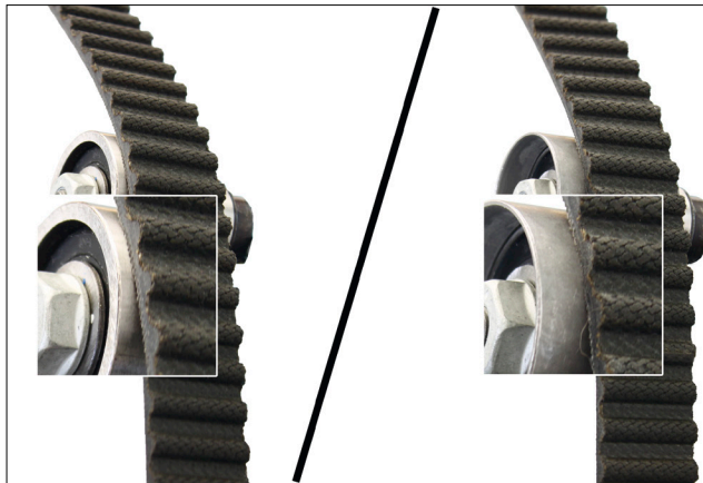
2. ábra: Balra az 532 0623 10 cikkszámú vezetőgörgő/ jobbra az 532 0349 10 cikkszámú vezetőgörgő
