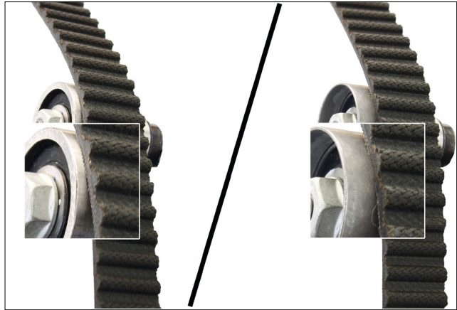
Kuva 2: Ohjainrulla 532 0623 10 (vasen)/ohjainrulla 532 0349 10 (oikea)
