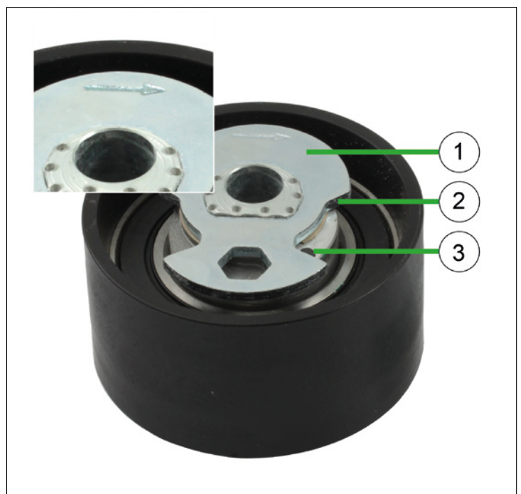
Figura 1: 531 0504 10 – Rullo tenditore semiautomatico
