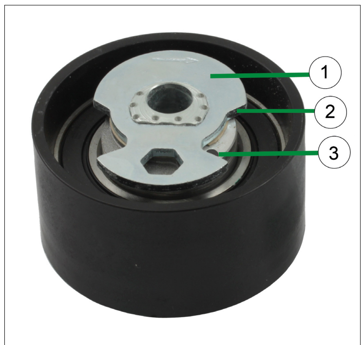
Slika 1: Kat.Br. 531 0504 10 – natezna remenica sa poluautomatskim sistemom natezanja
