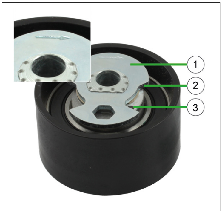
Photo 1 : 531 0504 10 – galet tendeur semi-automatique
