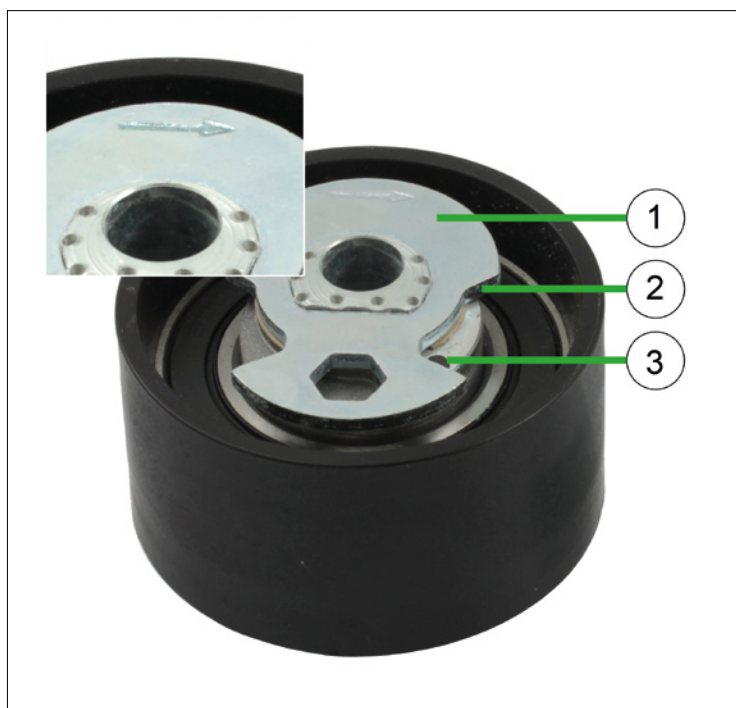
Figura 1: 531 0504 10 – Polea tensora semiautomática
