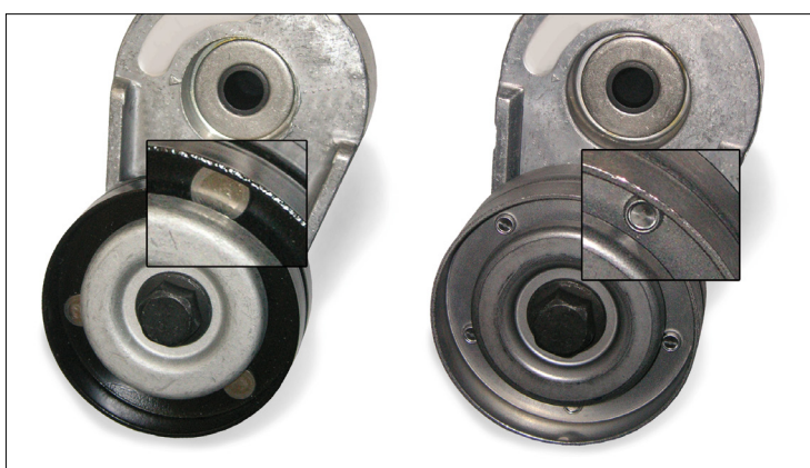
Slika 1: Natančen prikaz valjev v dosednji izvedbi (levo) in novi izvedbi (desno)
