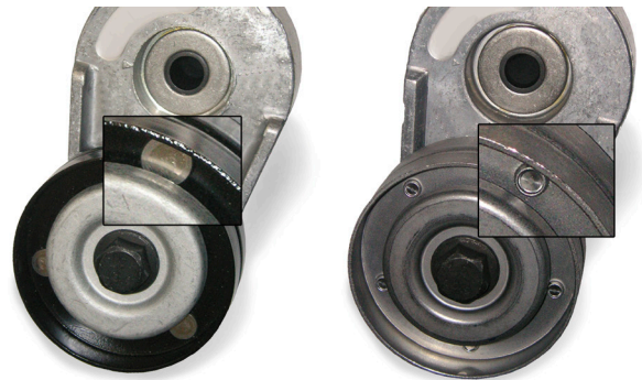
Εικόνα 1: Λεπτομερής όψη των τροχαλιών με τον προηγούμενο σχεδιασμό (αριστερά) και τον καινούριο σχεδιασμό (δεξιά)
